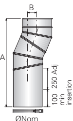
0-90° Adjustable Bend Extendable
