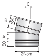
15° Bend
