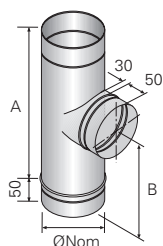
90° Tee
